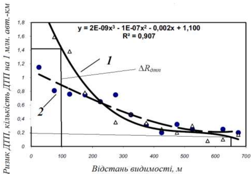
Рисунок 4 - Залежність показника ризику ДТП від відстані видимості у плані на багато смугових дорогах: 1 – з розподільчою смугою; 2 – без розподільчої смуги
