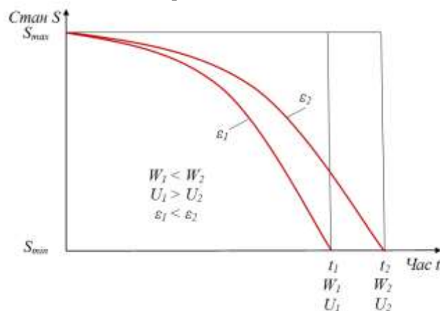
Рисунок 1 – Гіпотетичний вплив різних зусиль підрядника на стан елемента дороги
